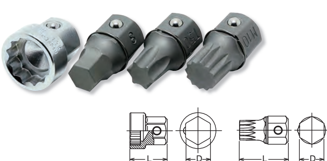
179B-12H Insert bit for the 145KD ratchet Einsatz-Bit für die Knarre 145KD Embout d'insertion pour cliquet 145KD
