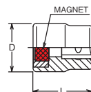
2120 Magnetic Head Magnetkopf Tête aimantée
