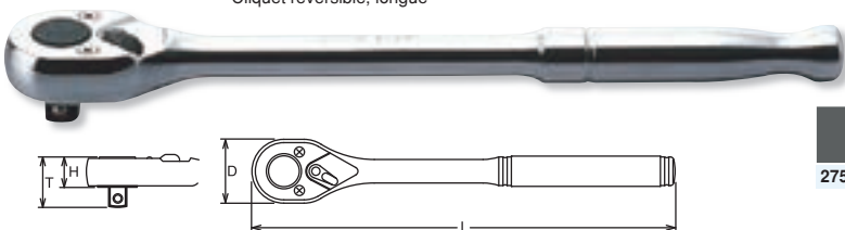
2753JB Reversible Ratchet with quick release button Knarre, verstellbar mit Verriegelungsknopf Cliquet, réversible avec bouton de débrayage
