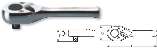
2753J Reversible Ratchet Knarre, verstellbar Cliquet, réversible
