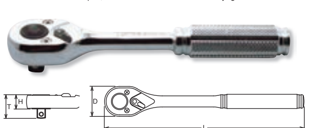
2753NB Reversible Ratchet with quick release button Knarre, verstellbar mit Verriegelungsknopf Cliquet, réversible avec bouton de débrayage
