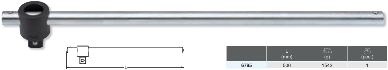
6785 T-Handle T-Griff Poignée coulissante
